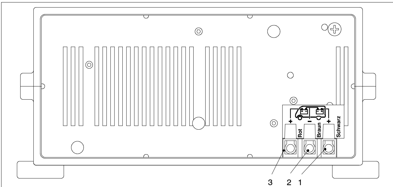
III. 5 Montage Bloc électrique EBL 119 (arrière)
