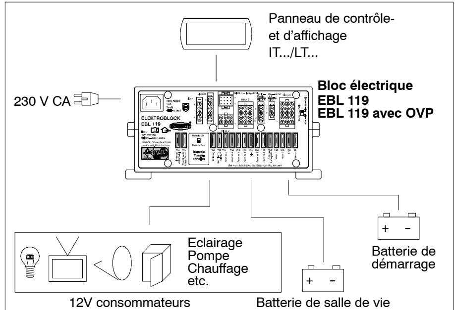
III. 2 Système d'alimentation en énergie à bord
